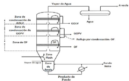
IMAGEN 4. ESQUEMA TECNOLÓGICO DE UNA COLUMNA DE DESTILACIÓN AL VACÍO
