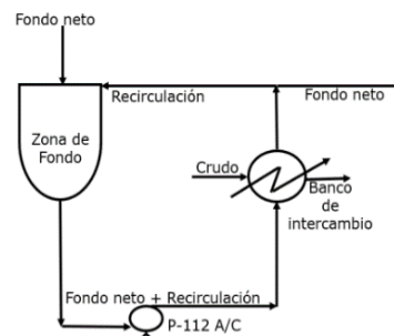
IMAGEN 6. FONDO DE UNA COLUMNA DE
