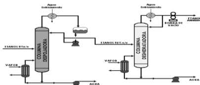
IMAGEN 7. DESTILACIÓN AL VACÍO
