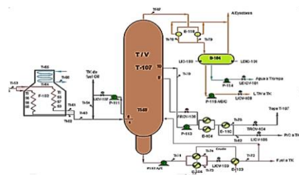
IMAGEN 5. FLUJO TECNOLÓGICO DE LA UNIDAD DE DESTILACIÓN AL VACÍO DE LA REFINERÍA NICO LÓPEZ.
