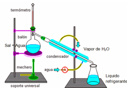
Imagen 2. Esquema del funcionamiento de la destilación al vacío
